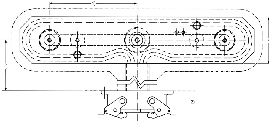
Ansicht X · View X · Vue X
