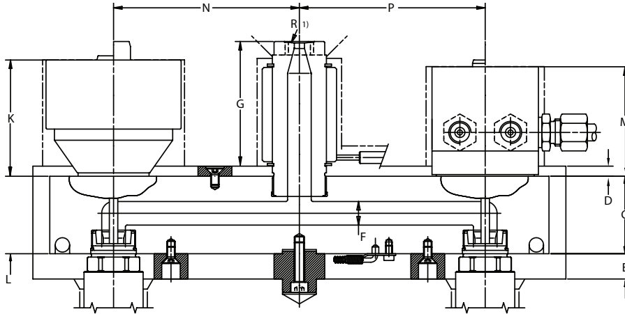
Ansicht X · View X · Vue X
